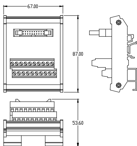
UB-10-ID16A
