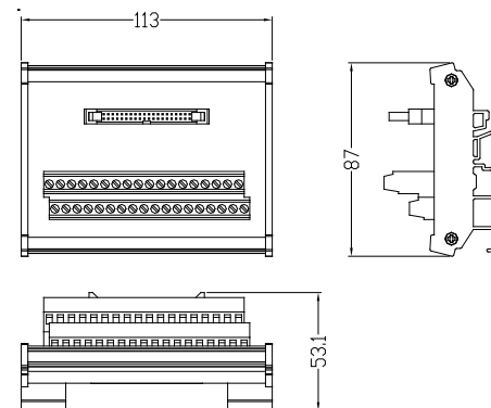
UB-10-OT32A
