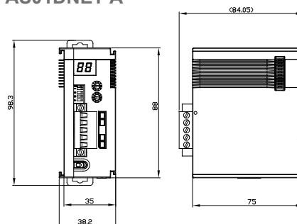
AS01DNET-A
