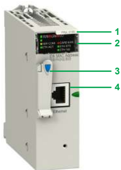
BMXPRA0100
