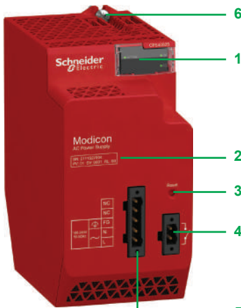
BMXCPS●●●2S
