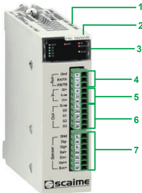
PMESWT0100
